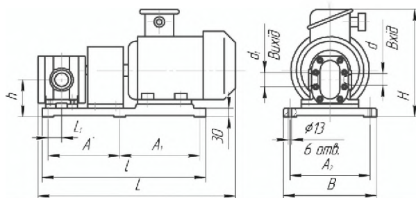
Габаритні і приєднувальні розміри насосних агрегатів БГ11-2
